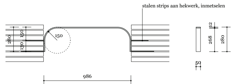
aanzicht hekwerk
