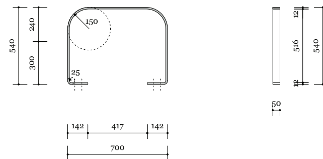
aanzicht hekwerk
